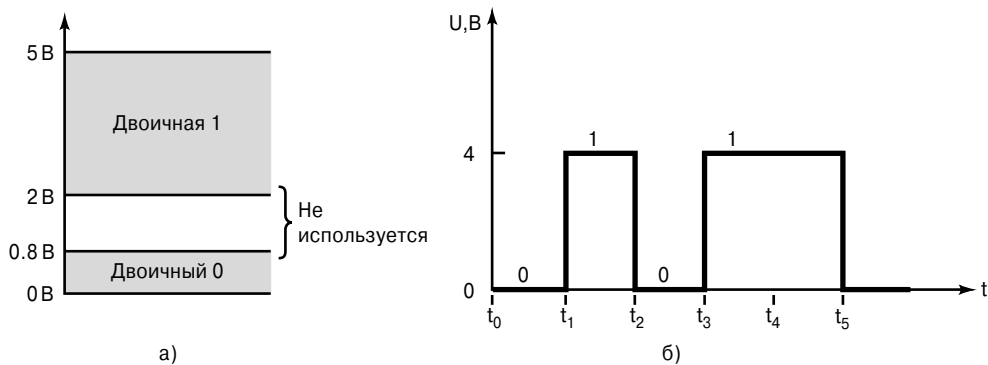
Рис. 1.7. а) Типичное распределение напряжений в цифровой системе; б) типичная временная диаграмма цифрового сигнала
