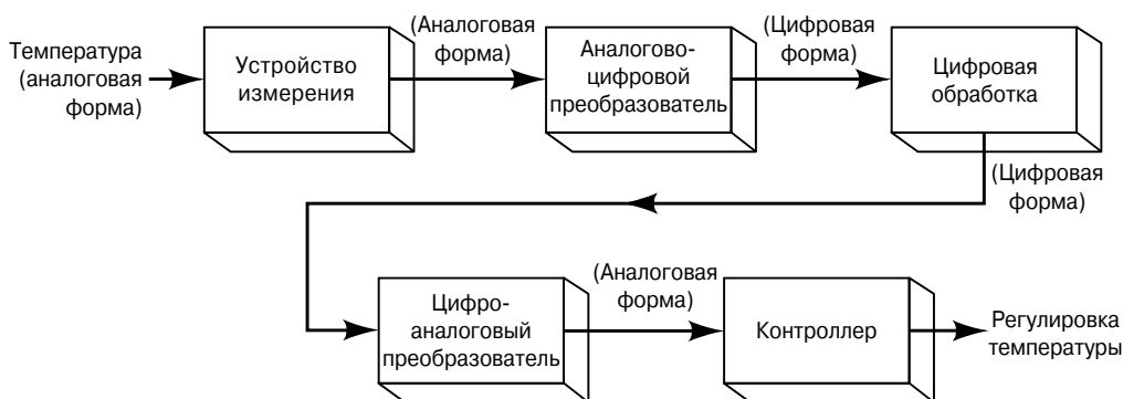
Рис. 1.1. Блок-схема системы контроля температуры, которая требует аналого-цифрового преобразования, для использования устройства цифровой обработки
