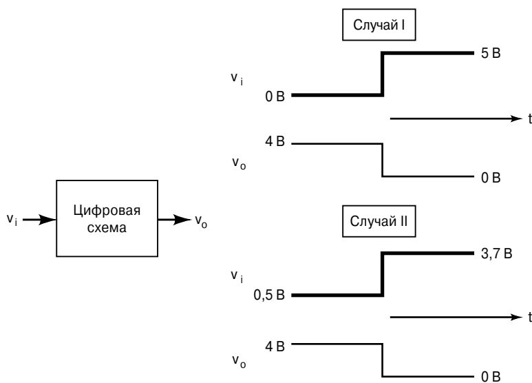
Рис. 1.8. Цифровая схема реагирует на двоичное значение входного сигнала (0 или 1), а не на фактическое значение напряжения
