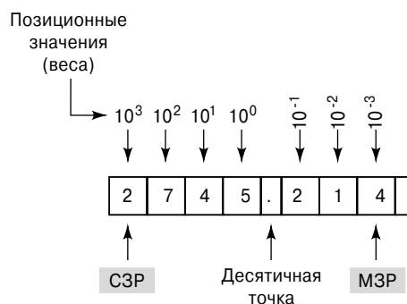
Рис. 1.2. Значение положения величины в десятичной системе как степени 10
