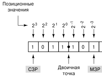
Рис. 1.4. Значения двоичных позиций в виде степеней 2
